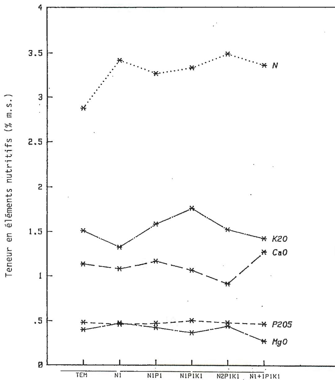
Fig. 22 Influence de la fumure minérale sur la teneur en substances nutritives des feuilles.
