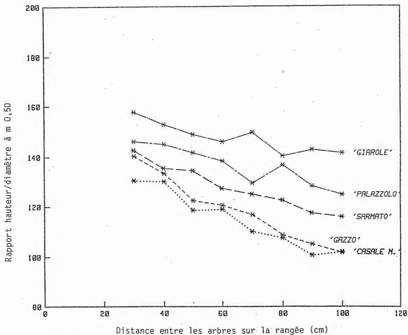
Fig. 4 Variations du rapport h/d des plants de peuplier âgés d'un an ( F_1 R_1 ) du clone LUISA AVANZO par rapport à la distance sur la rangée (distance entre les rangées m 2,20) et à la fertilité de la station.
